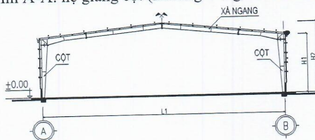
c) Mặt cắt 1-1
