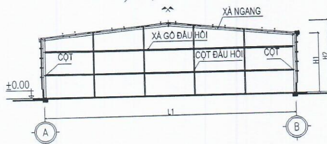
d) Hướng nhìn B-B: khung đầu hồi
