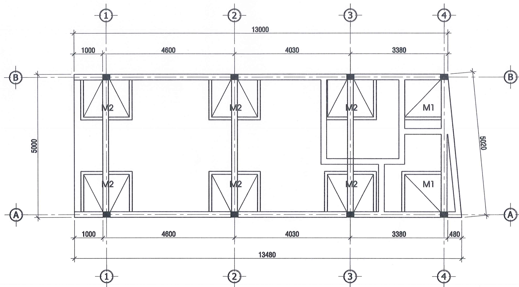
MẶT BẰNG MÓNG TL : 1/100
