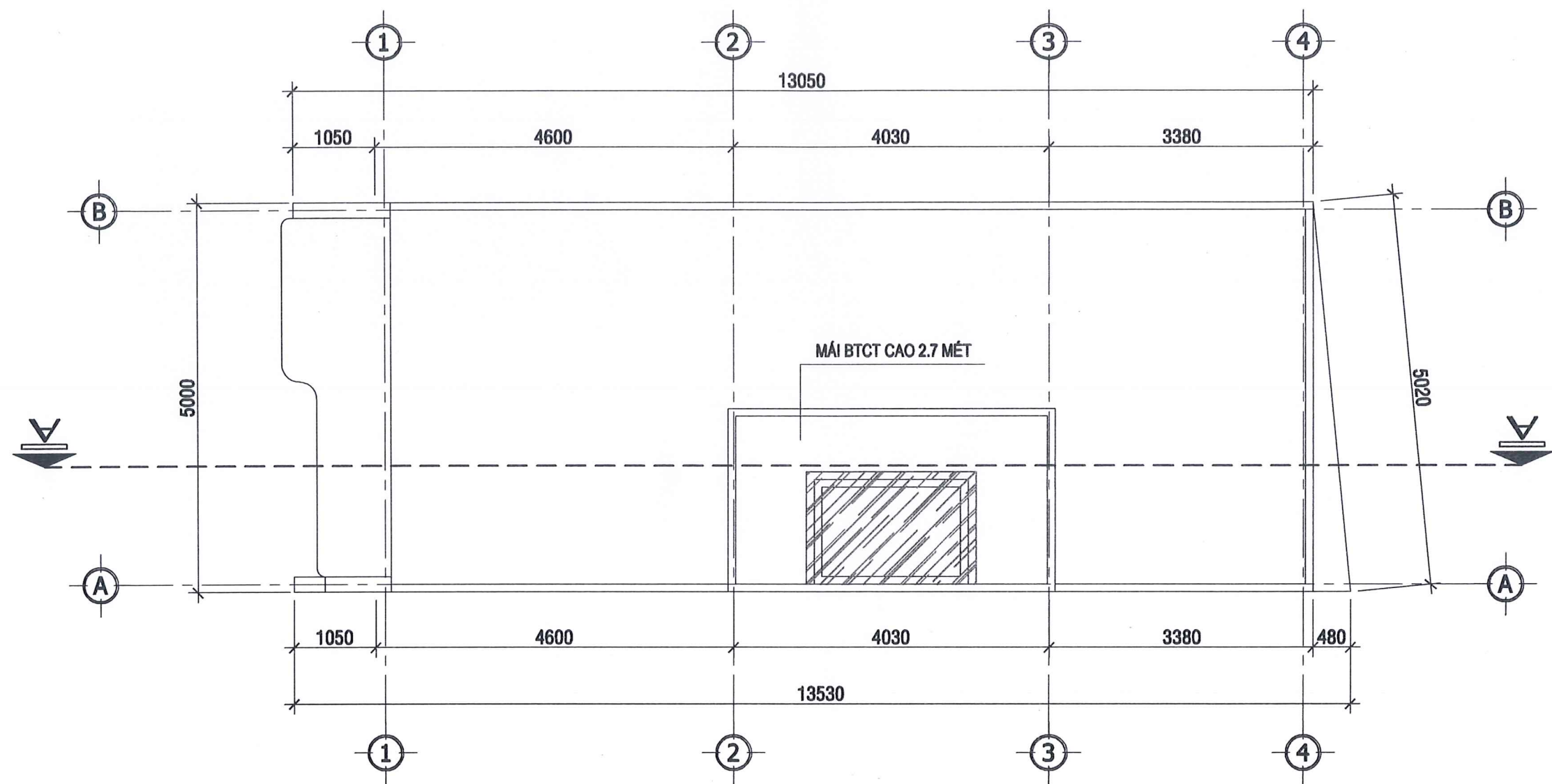
MẶT BẰNG MÁI TL : 1/100
