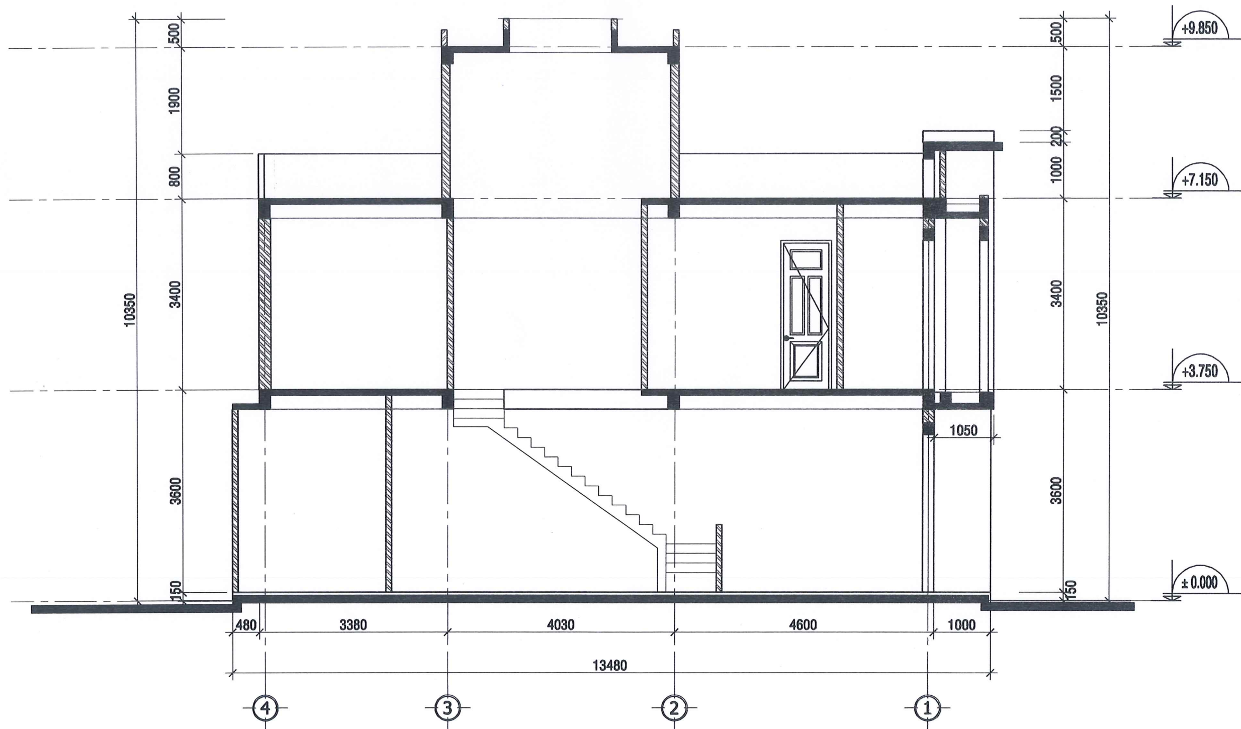
MẶT CẮT A- A TL : 1/100
