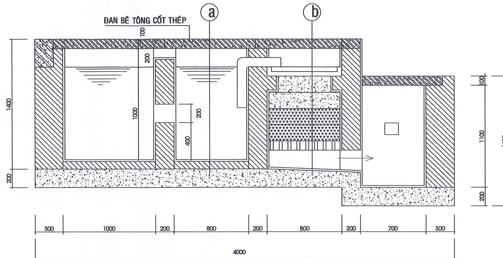
MẶT CẮT 1-1
