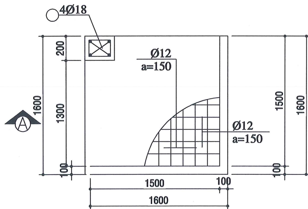
MB MÓNG M1 TL:1/50
