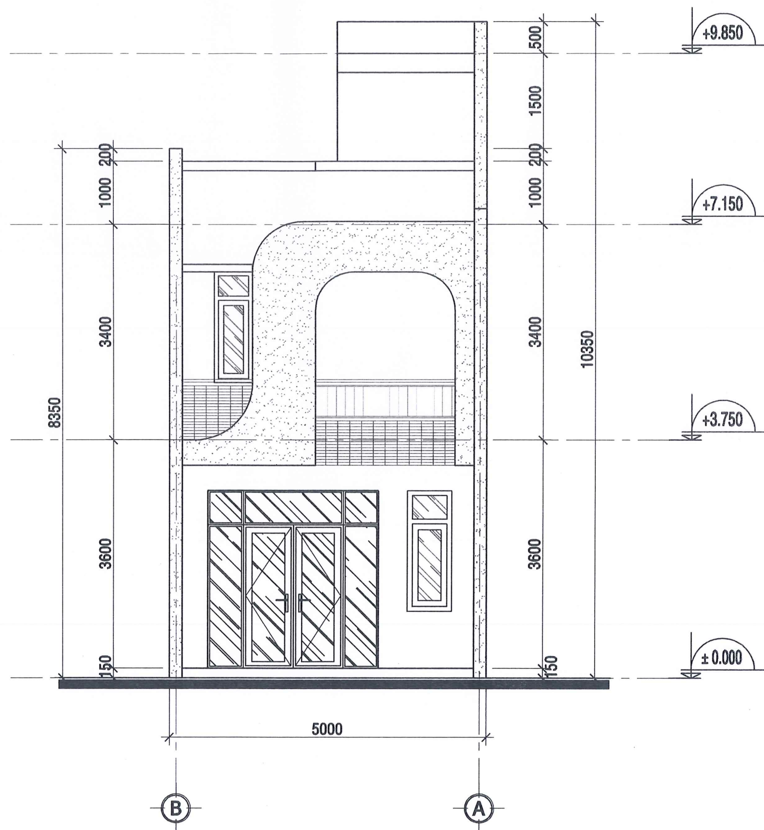
MẶT ĐỨNG CHÍNH TL: 1/100
